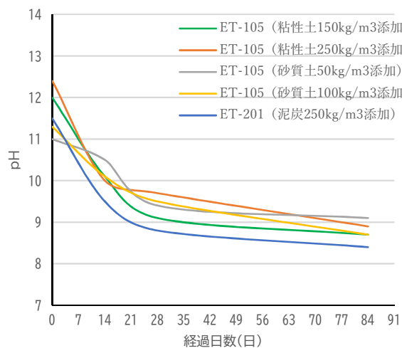
改良土に接した水のpH経時変化
